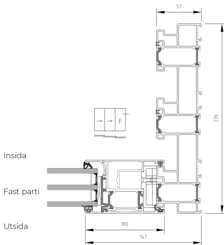
Fast parti från ovan
