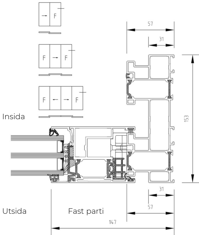
Fast parti från ovan
