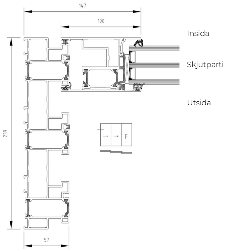
Skjutparti från ovan
