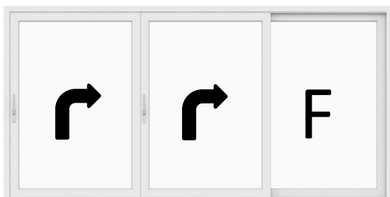
Schema E: 3-delat, två skjutdörrar bakom ett fast parti, 3-spår
