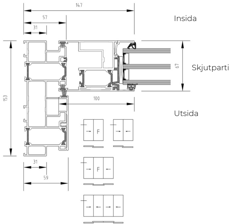
Skjutparti från ovan
